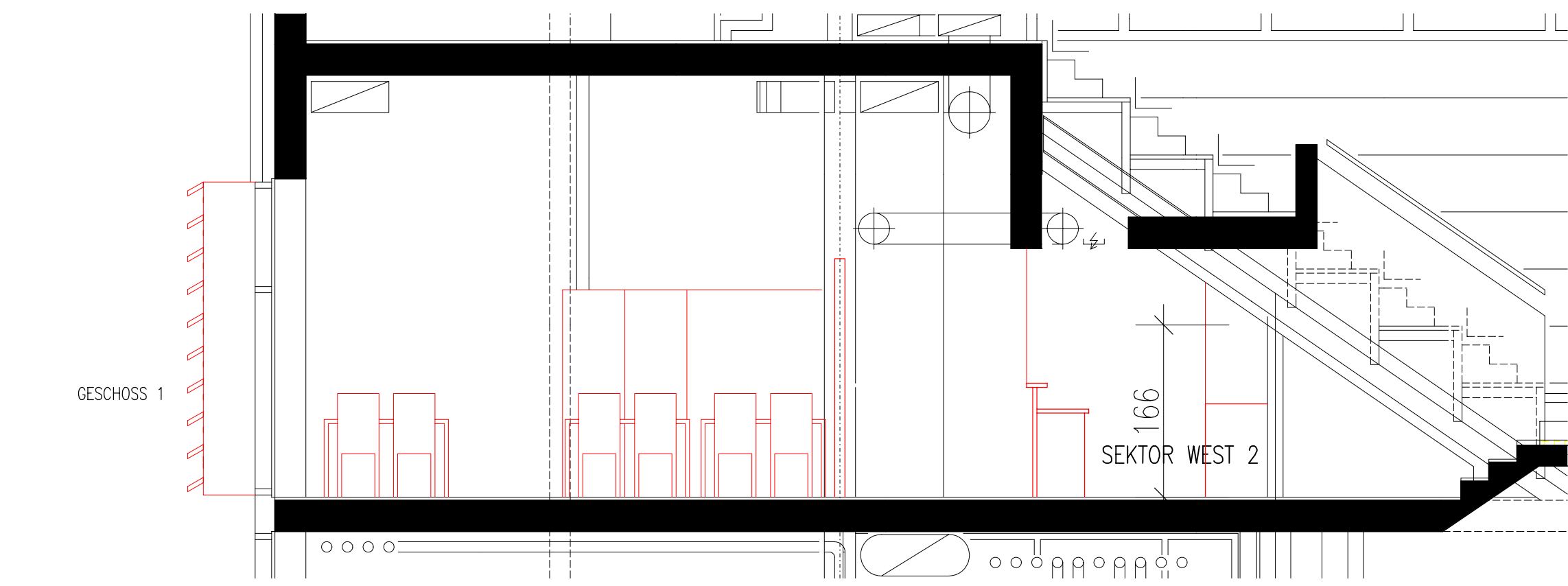
SNITT VARIANTE 1 MST.: 1:50
