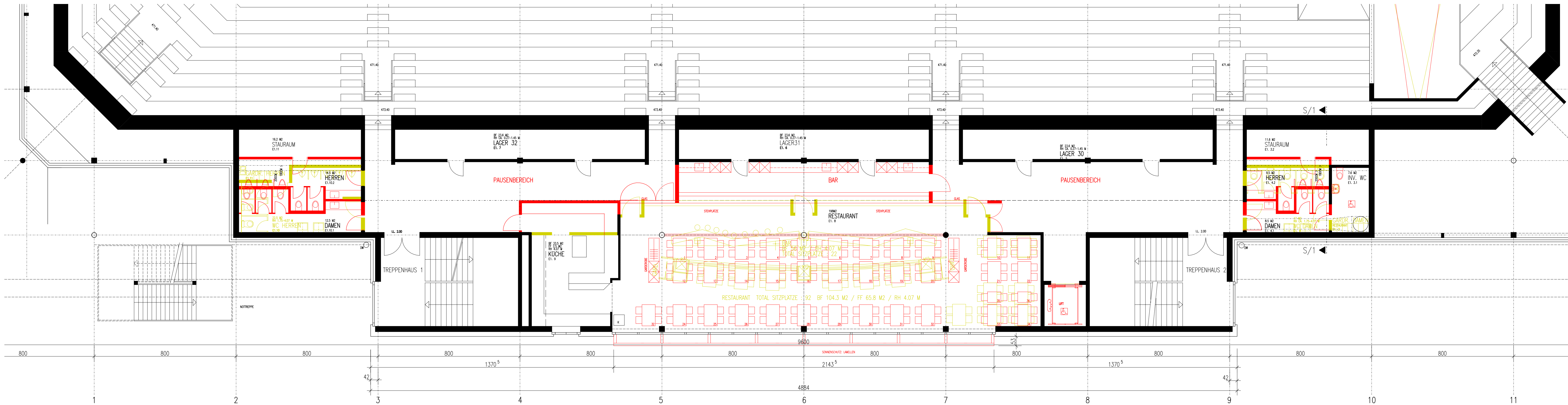
GRUNDRISS VARIANTE 1 MST.: 1:100
