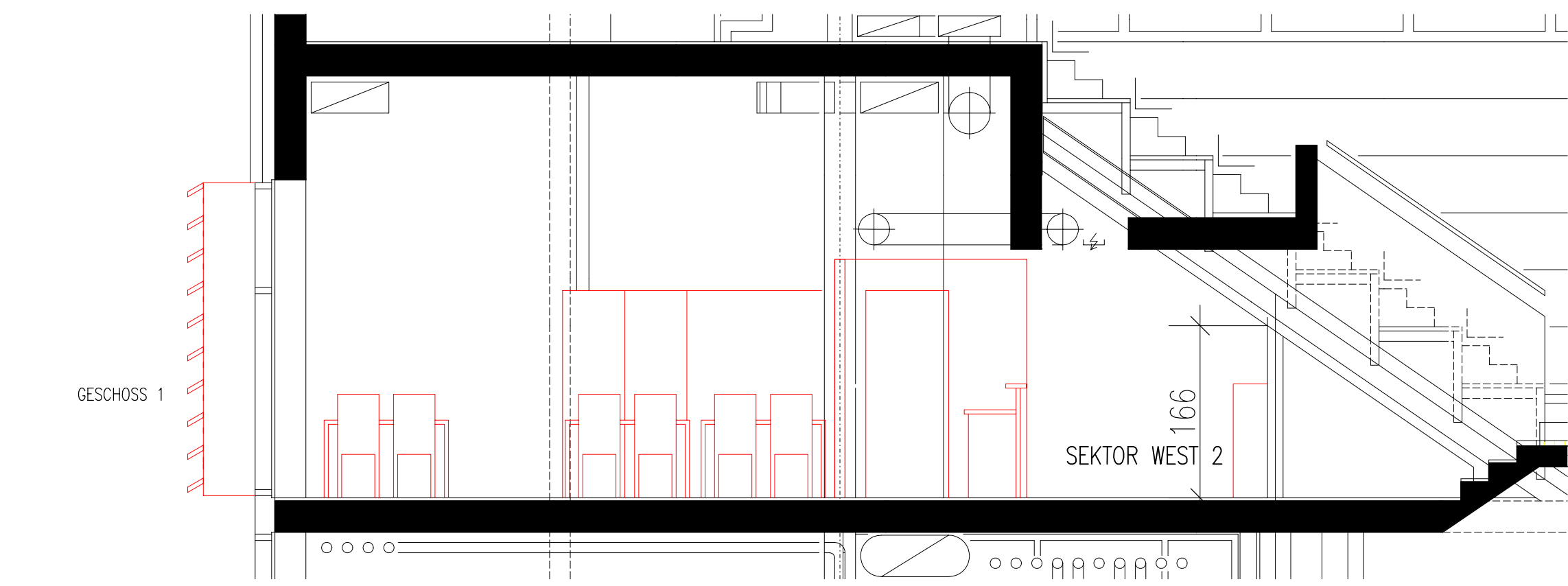
SNITT VARIANTE 2 MST.: 1:50
