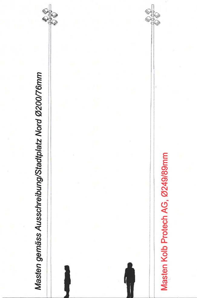
Abbildung 2: Beleuchtungsmasten H=15.00m, Vergleich Durchmesser
