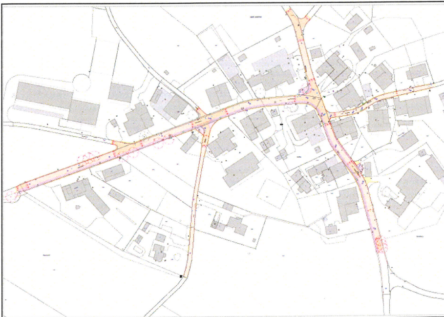
Oberflächengestaltung Gerlisberg Dorf, Kloten
