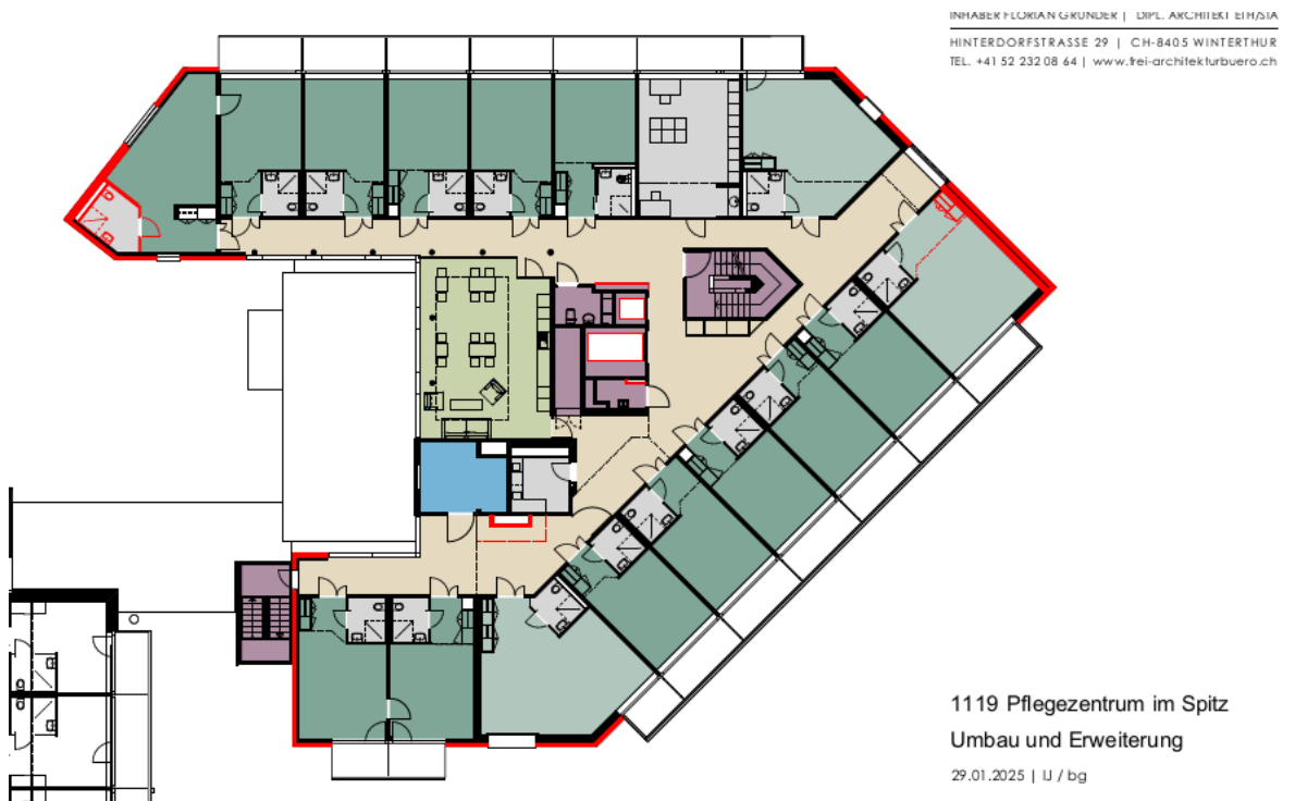
Grundriss 2. – 4. Obergeschoss, bestehende Zimmer / Stübli (grün), Erdbebenertüchtigung Eckzimmer, neue Fassade Brandschutz (rot)
