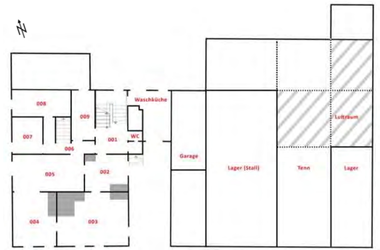
Abb. 34: Schematischer Grundriss Erdgeschoss. Bearbeitung IBID.
