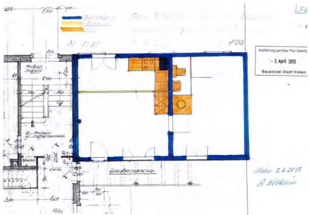
Abb. 121: Umbau Verbindungsbau im 1. Obergeschoss, 2013. Bauamt Stadt Kloten.
